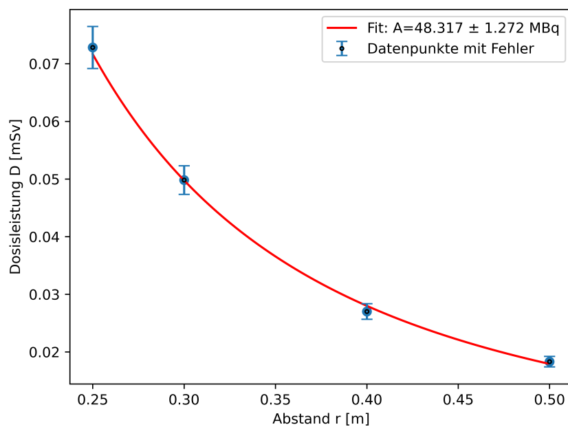
(b) Cs-137 Referenzquelle (Quelle Nr. 8)
