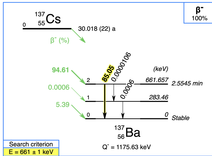
Abbildung 2.4.: Das Zerfallsschema von Cs-137 zu Ba-137. Das relevante Energieniveau bei E_2 = 661,657 keV ist mit der zugehörigen Emissionswahrscheinlichkeiten gelb eingefärbt. [11]
