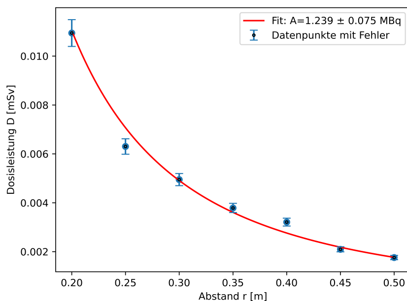
(a) Co-60 Referenzquelle (Quelle Nr. 3)
